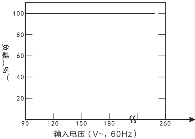
ZZZ-WAX75-K机型静态特性
